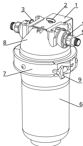
Рис. 1. Схема установки корпуса водоочистителя
