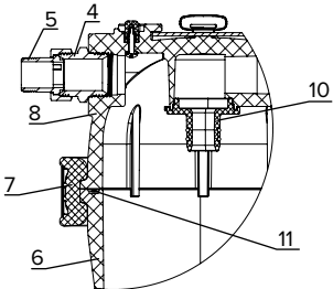
Рис. 2. Разрез по месту соединения коллектора и стакана
