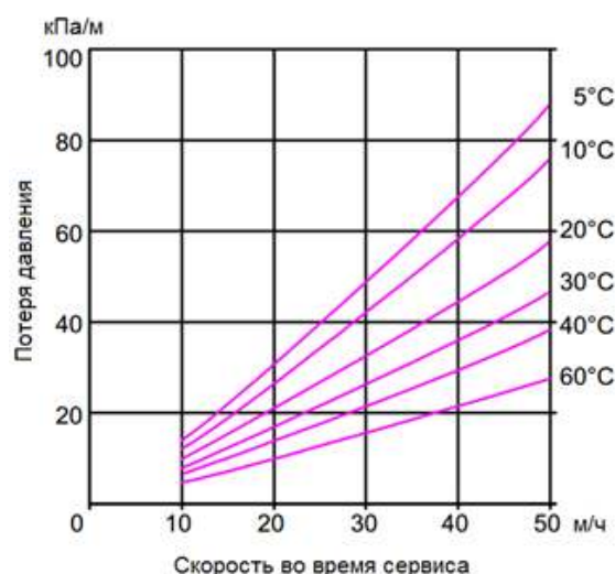
Рис. 2. Потери давления
