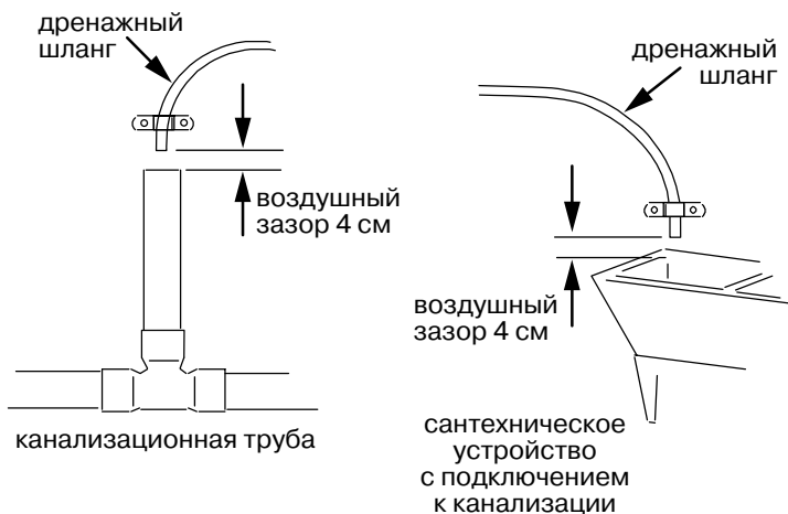
Рис. 3. Подключение дренажа
