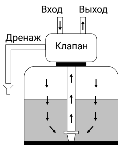
Рабочий режим
