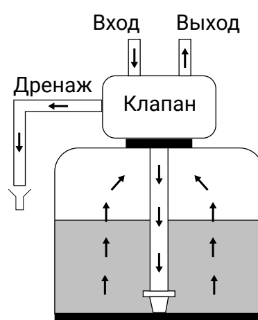
Обратная промывка
