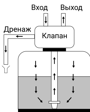
Прямая промывка
