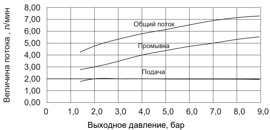
Инжектор 2 (Синий)
