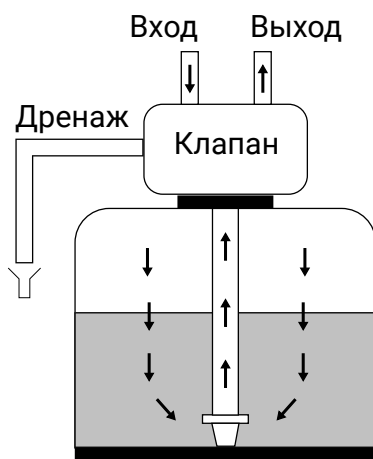
Рабочий режим
