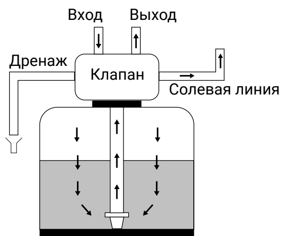
Заполнение бака-солерастворителя
